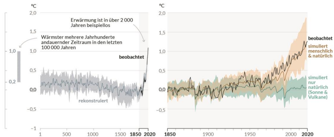
Abbildung 2-2: Menschengemachte Erwärmung seit der Industrialisierung
